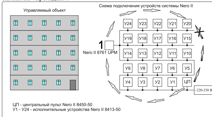
Рисунок 5 Пример реализации режима «ретранслятор» по сети ~220-230 В
