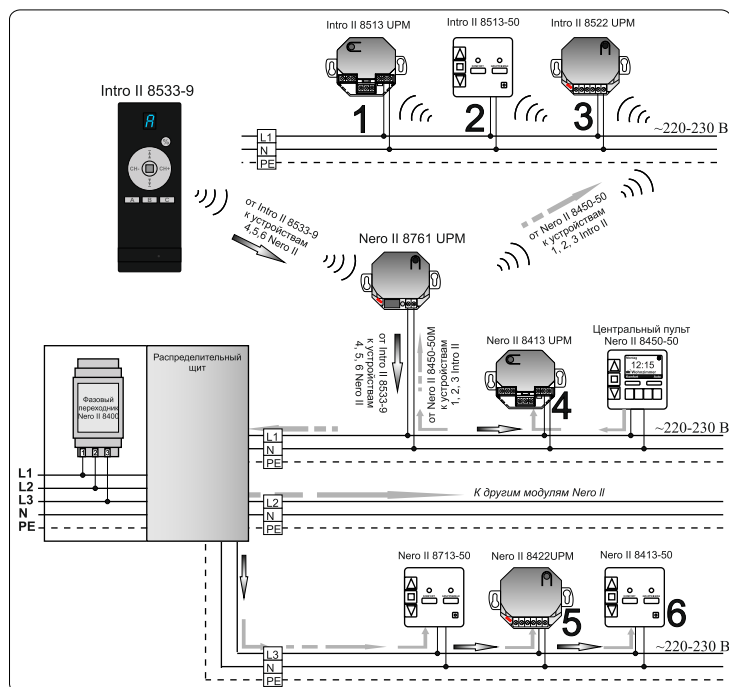
Рисунок 1 Принцип действия устройства Nero II 8761 UPM
